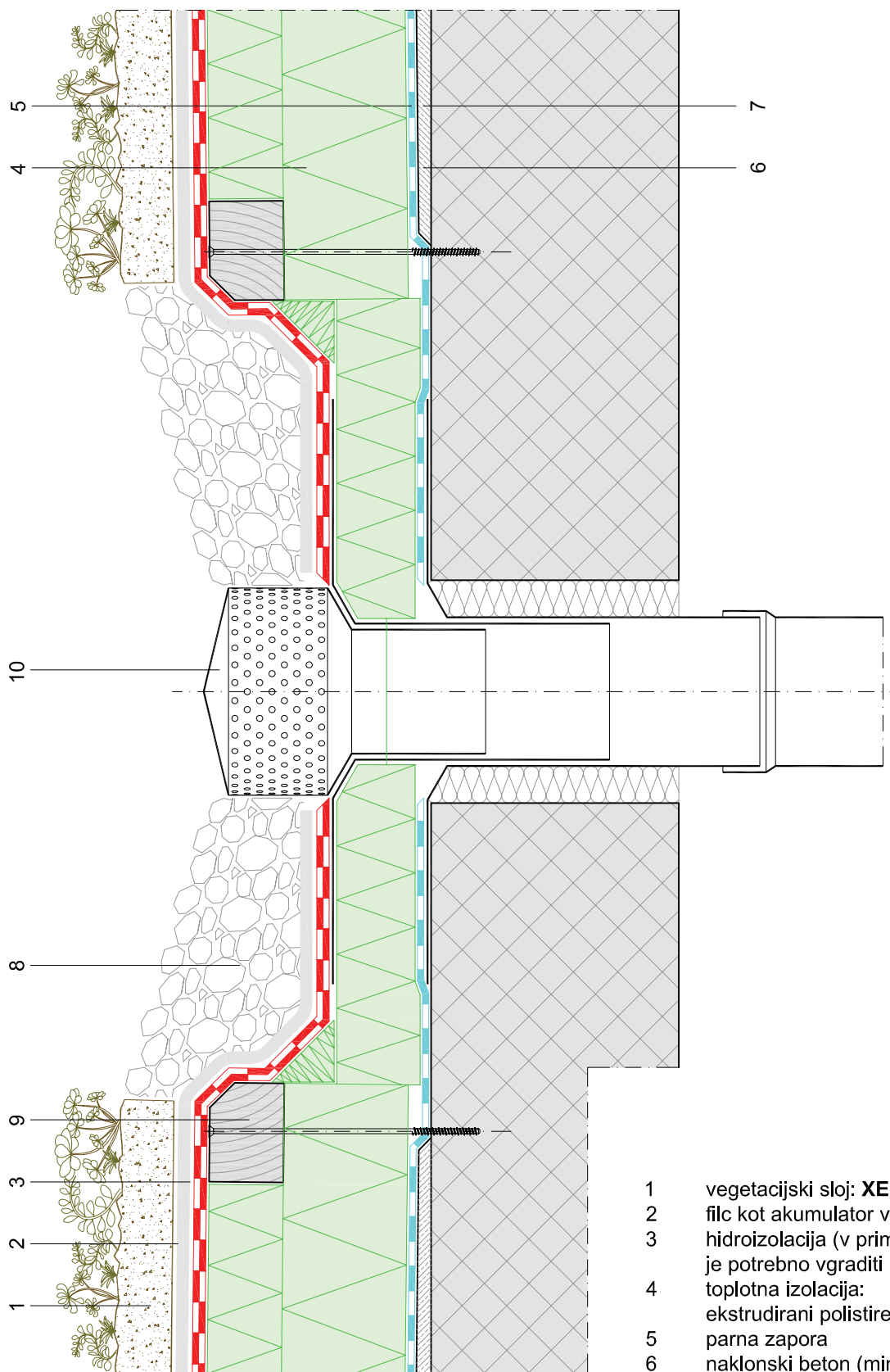
detajl 3.3 - masivna topla streha - klasični odtok
