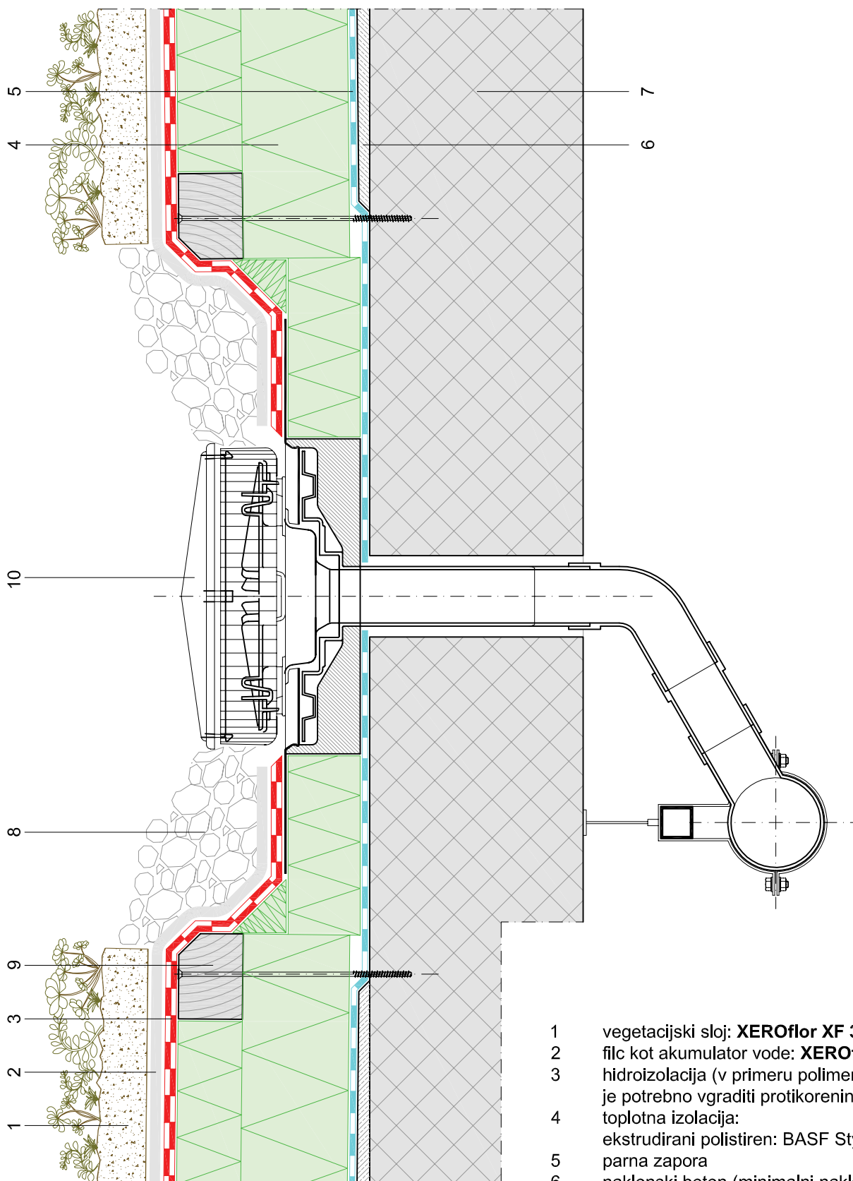
detajl 3.4 - masivna topla streha - odtok Pluvia
