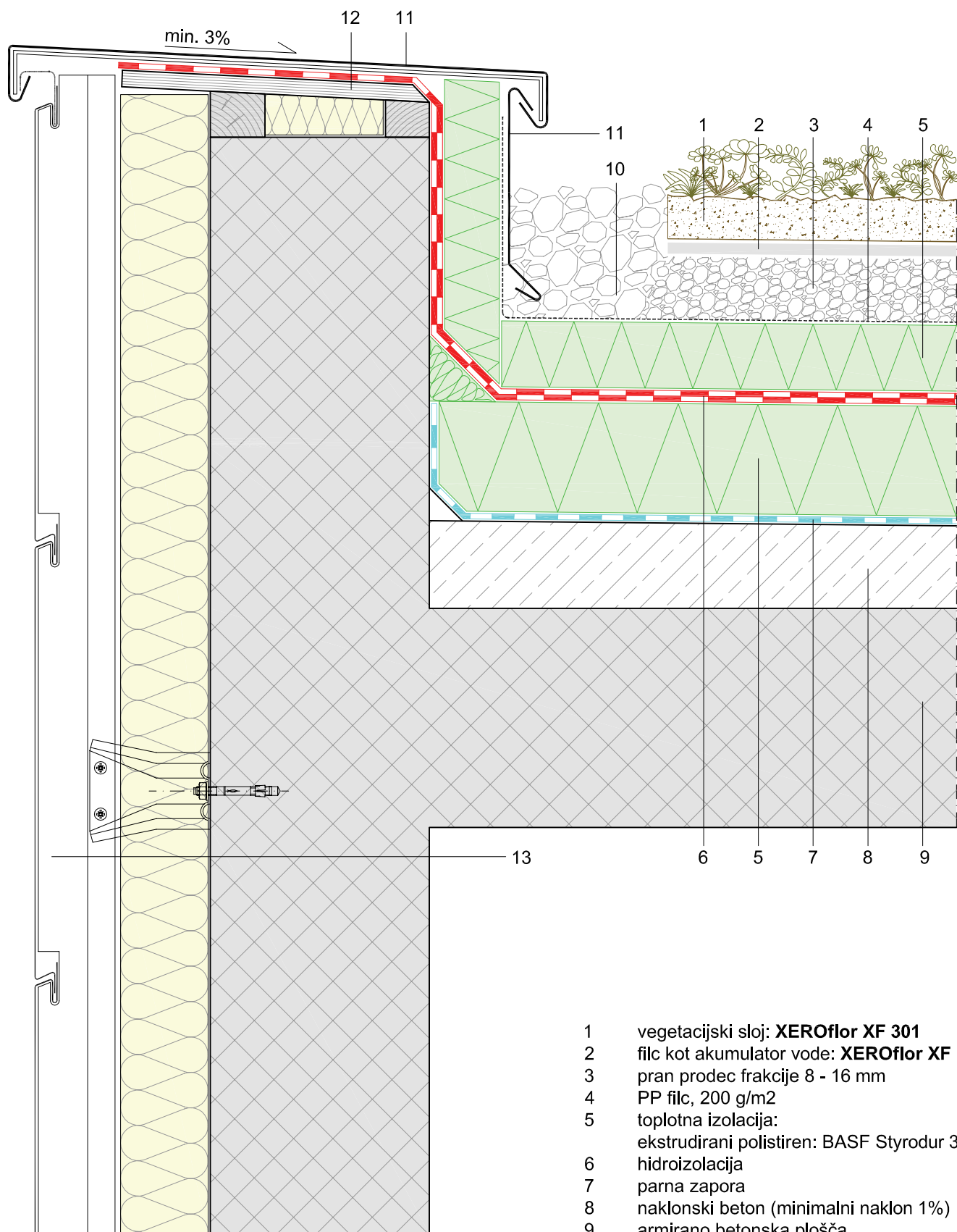
detajl 1.2 - kombinirana obrnjena streha - strešni venec
