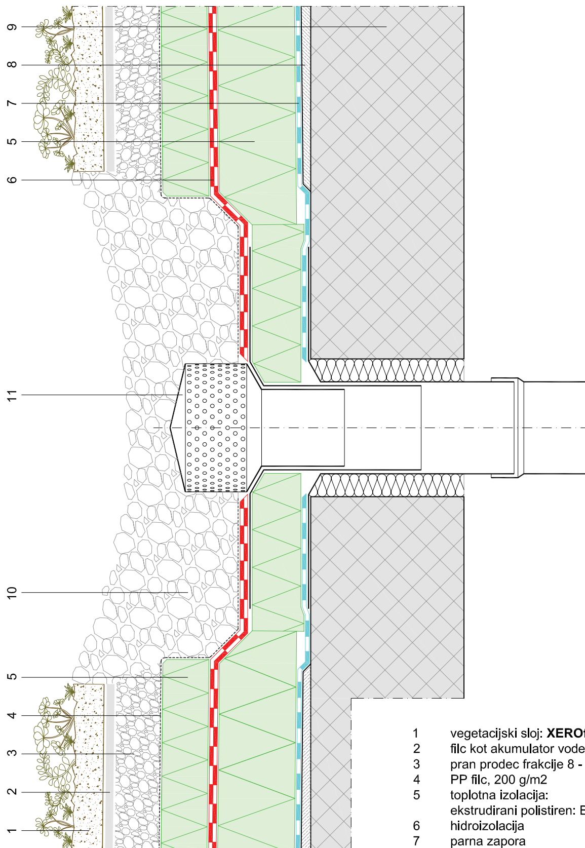
detajl 1.3 - kombinirana obrnjena streha - klasični odtok
