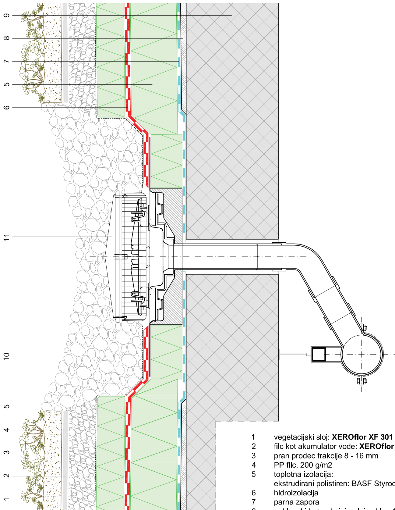
detajl 1.4 - kombinirana obrnjena streha - odtok Pluvia
