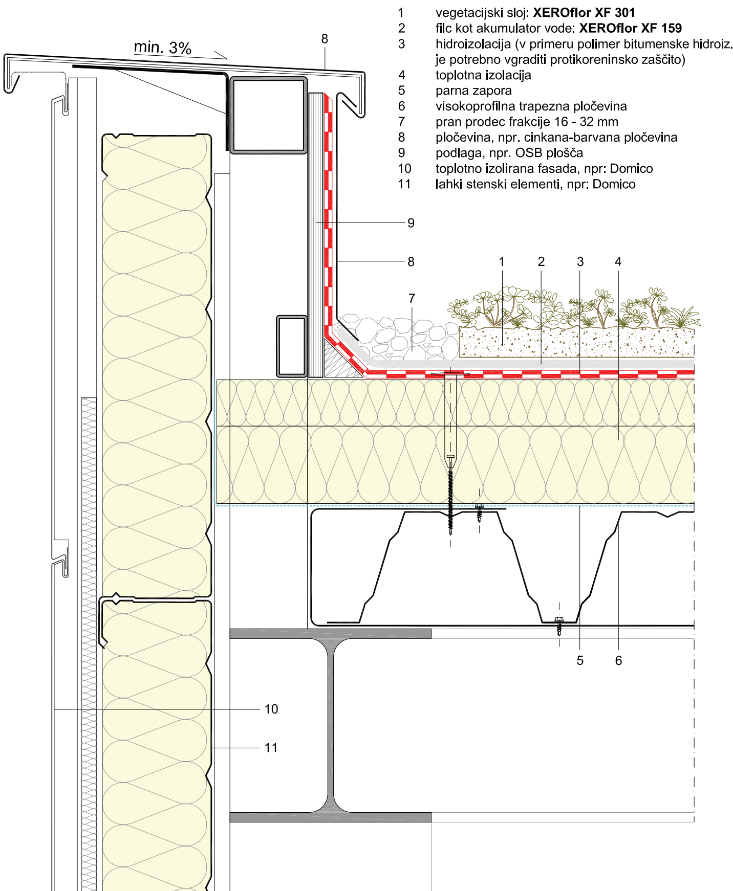
detajl 2.2 - lahka topla streha - strešni venec
