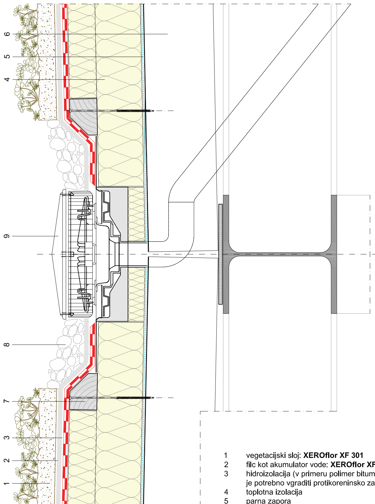
detajl 2.4 - lahka topla streha - odtok Pluvia
